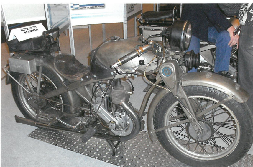
En smuk Neander mc fra slutningen af tyverne (lighed med samtidige Opel motorcykler er påfaldende, men de var også lavet på licens fra Neander).
