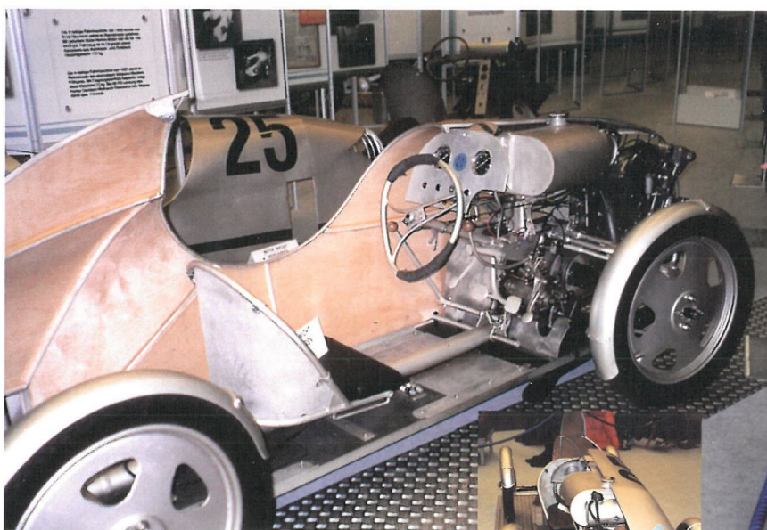
Et afsnit af udstillingen behandlede interessante småkøretøjer fra tyverne og tredverne på motorcykelbasis. Her en Neumann-Neander Fahrmaschine – bemærk centralrørschassiseet
