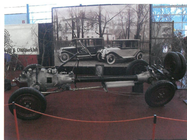
Den tyske Tatra-klub havde gjort Hans Ledwinkas chassis-konstruktion med centralrør til det i bogstaveligste forstand bærende princip på sin klubstand.
