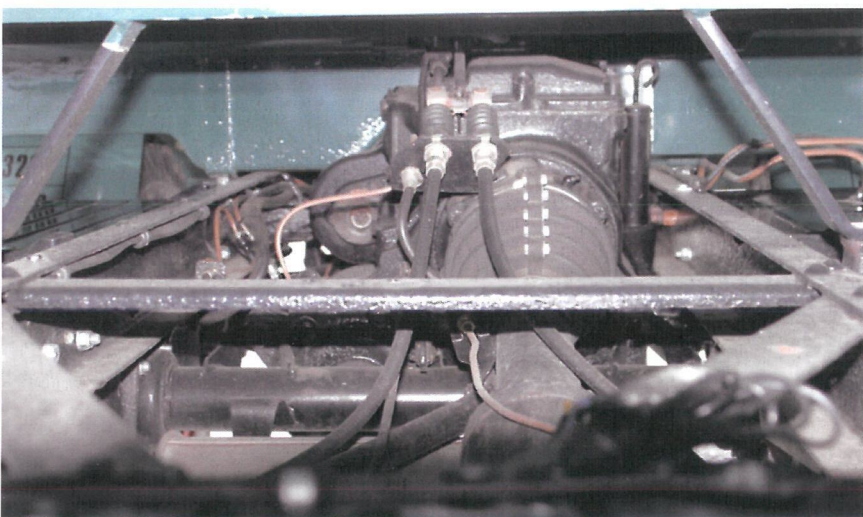
Et kig under maven, man ser chassisets langsgående vanger, fordelergearkassen med gummibælgen lidt th. i billedet med håndbremsekabler og bremserør - bemærk pejlestokken til kontrol af gearkassens oliebeholdning.
