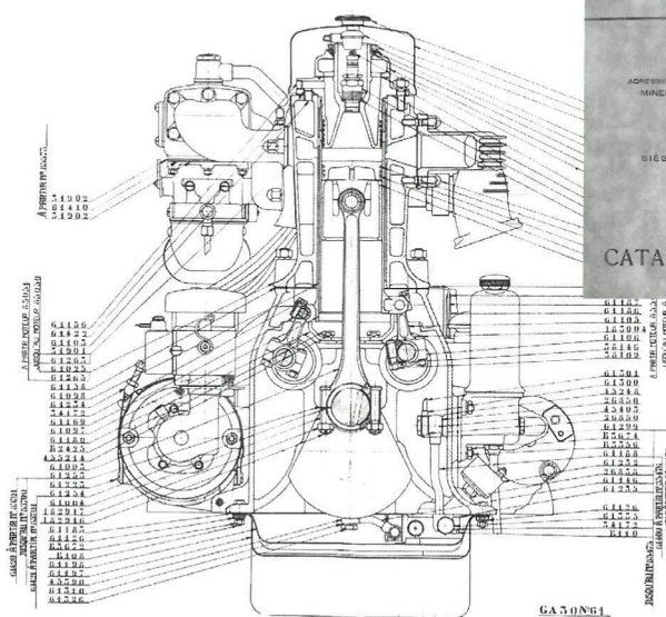
Moteur coupe transversale, (par un cylindre) Chassis type Court et Long.
