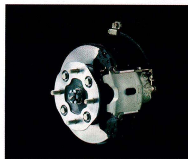
4. Store skivebremses foran og tromlebremses bagi er servoforstærkede. Bremsesystemet er et diagonalt 2-kredssystem.
