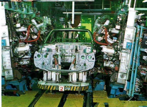
Karosseriet svejdes i 130 punkter med præcise maskiner.
