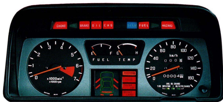
1. Målere, kontrol- og advarselsindikatorer er let at overskue.
