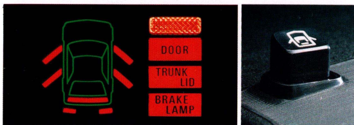
2. En sikkerhedsindikator med tilhørende chekknep gør Dem øjeblikkelig opmærksom på ikke-lukkede døre og/eller defekte bremselys.
