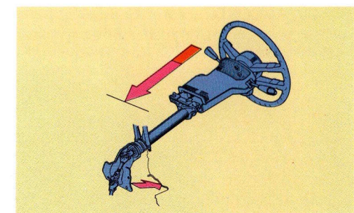
17. Ratstammen er sammenskydelig.
