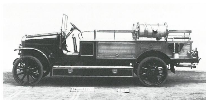
Autospritze, Typ Bayern, Baujahr 1921 Vehicle mounted fire extinguisher, type Bavaria, year of manufacture 1921 Pompe de véhicule, type Bavière, année de construction 1921 Bomba de vehículo, tipo Baviera, año de construcción 1921
