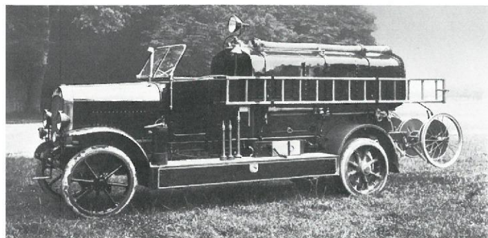
Tankspritze für Rumänien, Baujahr 1924 Fire-fighting water truck for Rumania, year of manufacture 1924 Pompe automobile à réservoir pour la Roumanie, année de construction 1924 Bomba montada sobre el tanque para Rumania, año de construcción 1924
