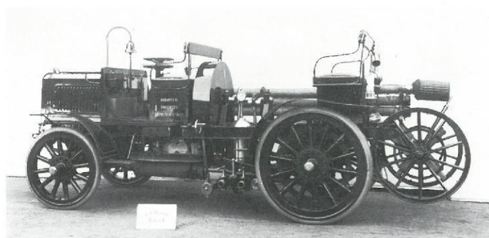
Benzin-Autospritze für Budapest, Baujahr 1903 Gasoline operated car water pump for Budapest, year of manufacture 1903 Pompe à moteur de véhicule pour Budapest, année de construction 1903 Motobomba de vehículo para Budapest, año de construcción 1903
