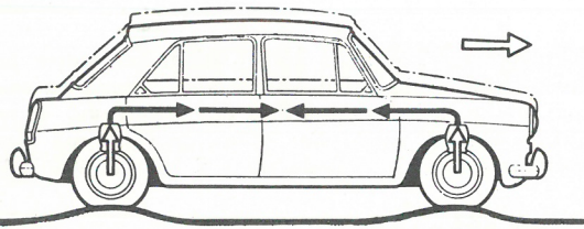
Affjedringen bliver stivere, hvis for- og baghjul løftes af ujævnheder samtidig = Behersket lodret karrosseribevægelse (hop)
