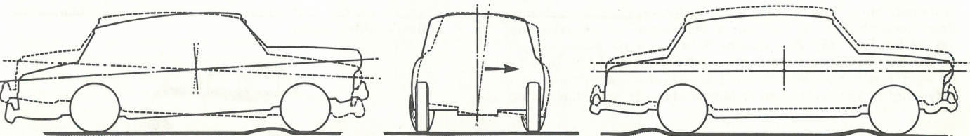
NIKSVINGNINGER – karrosseriet nikker om sin tværakse
