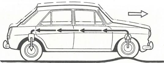
Bagvognen hæver sig, når forhjulene kører over ujævnheden = Ingen niksvingning
