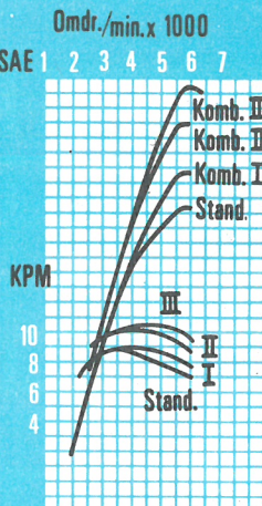
Effektdiagram for AUSTIN 1100 mk II
