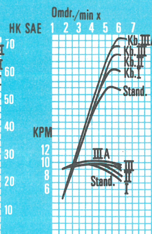
Effektdiagram for Austin 1300 mk II
