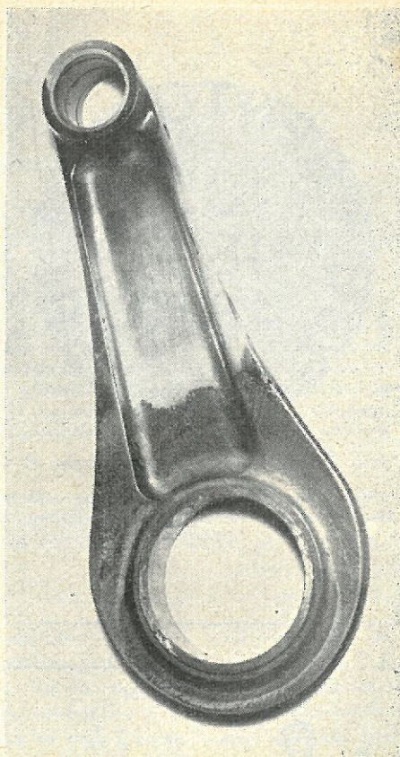
Også de mekaniske elementer sætter en vis grænse for tuningens omfang — for motoren skulle jo gerne holde. Her er plejlstangen fra en Norton Manx. Vi kan dog lære af højglanspoleringen, hvilket senere skal omtales.
