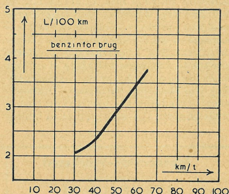
Husqvarna's laveste benzinförbruk ligger omkring 30 km/t, og fra 40 km/t stiger forbruget efter en fuldstændig ret linie.
