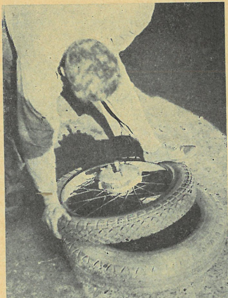
Så vender vi hjulet om og træder den anden kantråd på plads. På værkstedet bruger vi næsten altid en hammer, men sådan een kører man jo ikke rundt med. De fleste motorcykle-dæk kan man træde ned hele vejen rundt, men hvis det kniber på det sidste stykke, kan De blade om til næste side...
