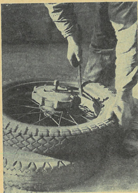
...og med dækjernet vipper vi den ene side af dækket ind over fælgen — det er uhyre let og kan næsten gøres med de bare hænder. Vi begynder modsat ventilen.
