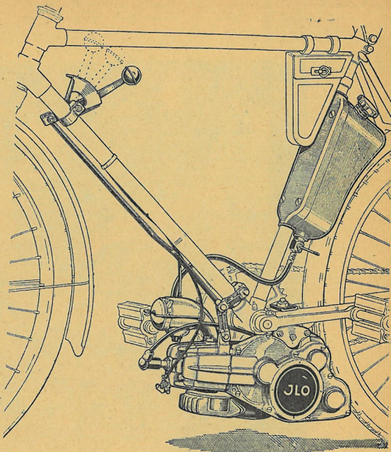
Ilo F 48 bespændes direkte under kranken, og der skal ikke foretages ændringer på cyklen.
