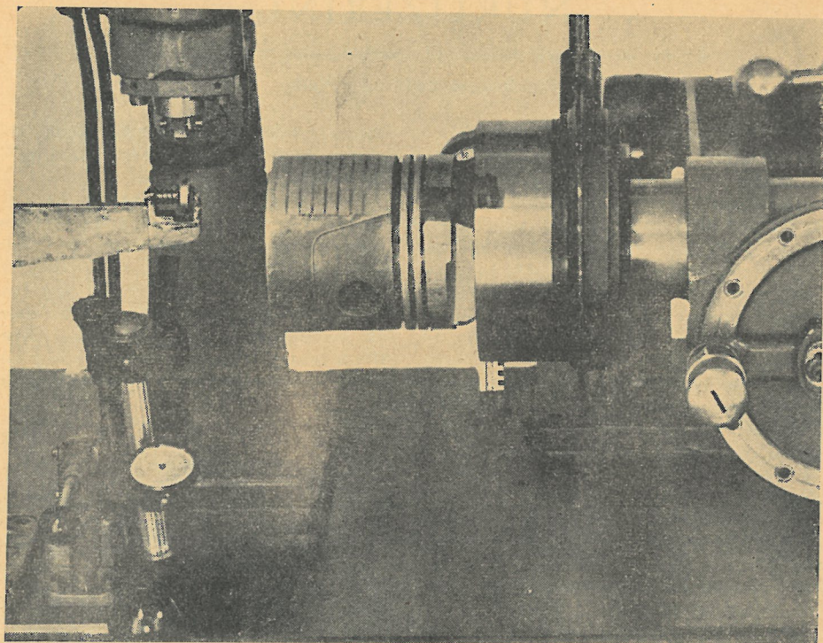
Stemplet spændes op i en specialmaskine, og mønstret presses i ved hjælp af komprimeret luft.
