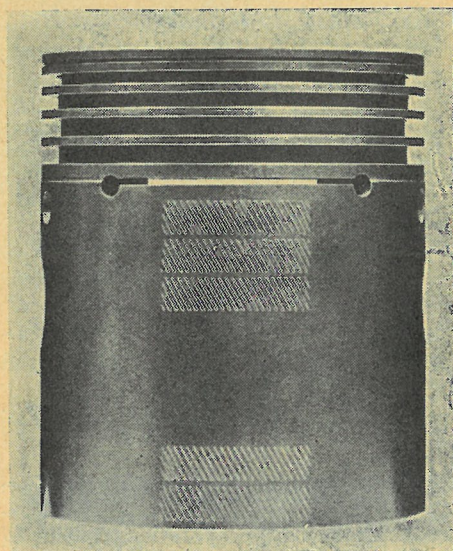
Ved nurlizeringen indpreses et mønster på stemplets bæreflader.
