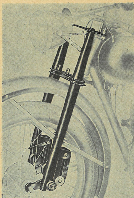
Husqvarna har en særpræget forhjulsophængning bestående af en svinggaffel med gummibånd som fjedrende element. Gummibåndene, der har en kraftig egendæmpning, overflødig gør brugen af støddæmpere.
