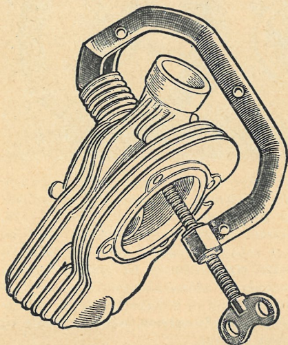
En skruevinge til afmontering af ventilerne er et uundværligt stykke værktøj, når man skal vedligeholde og reparere en fire-takt motor.
