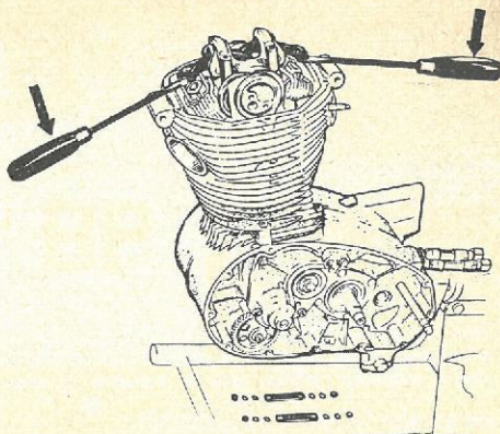
Når møtrikker, skiver og lasker til legebukkene er fjernet, løfter man hele knastakselhuset af. Et par skruetrækkere eller lignende bruges som vægtstænger med den ene ende anbragt under vippearbene.
