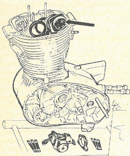
Ekscentrikken mærkes med et tydeligt kryds, inden den fjernes.
