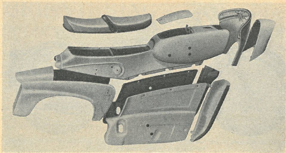
Pladekonstruktionen til Ariel Leader. Som det ses, er rygraden, der består af „benzintanken" og den øverste del af bagskærmen med konsol for dobbeltsædlen, udformet som et centralrør.
