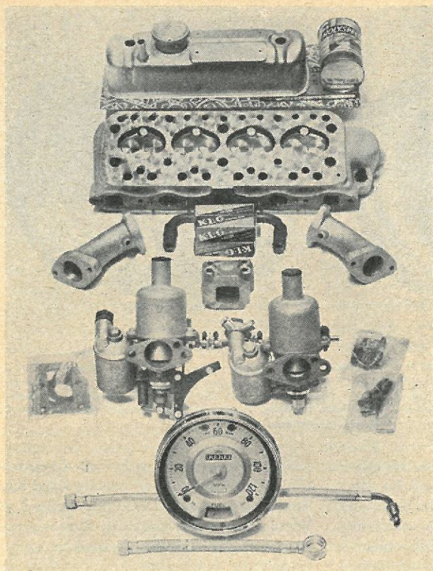
Delene til et Speedwell tuningsæt beregnet for en BMC motor. Foruden det specielle topstykke er der specielt indsuigningsmanifold beregnet til to SU karburatorer. I forgrunden ses et universal kontrolorgan med speedometer, kilometertæller, fire kontrollamper og benzinstandsmåler. Dette topstykke med de to karburatorer vil foruden en forbedret accelerationsevne også give forbedret økonomi ved konstante hastigheder, men i bytrafik vil benzinforbruget sandsynligvis stige, når den store accelerationsevne til stadighed udnyttes.
