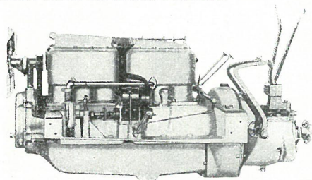
Den ideelle, 6 cylindrede moderne Motor, kraftig, lydøs, renlig og kompakt. Bemærk hvor smukt hver enkelt Del er arrangeret, praktisk og let at komme til.
