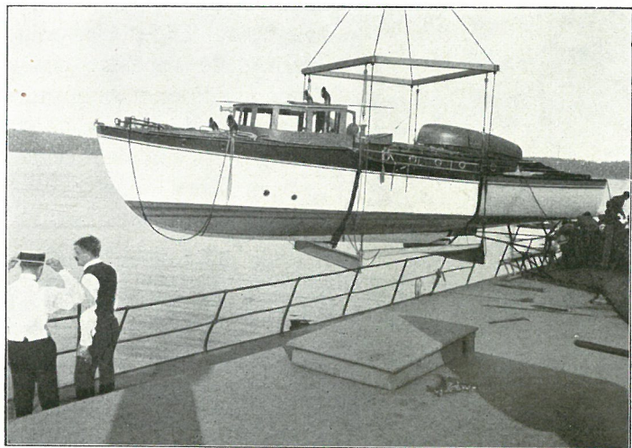
Udenskærskrydseren „Penta IV“, bygget 1910 til Konkurrencen Stockholm—Göteborg, ophængt til Vejning (Bestemmelsen af D = Deplacementet i Formlen).
