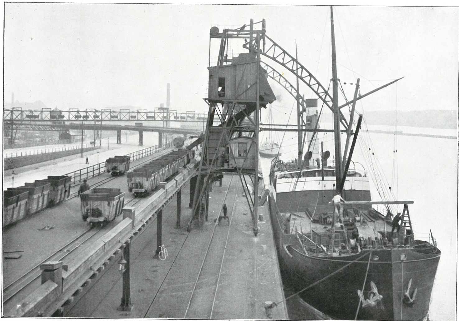
Fig. 10. Belysningsvæsenets Kraner og Kabelbane paa Kalvebodbryggen.
