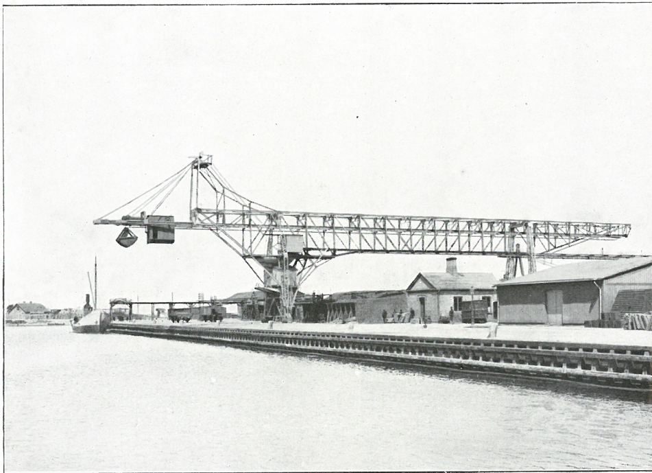
Fig. 8. Kulkran i Malmö Havn.
