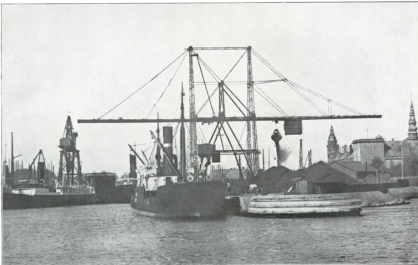
Fig. 7. Kulkran i Helsingør Havn.
