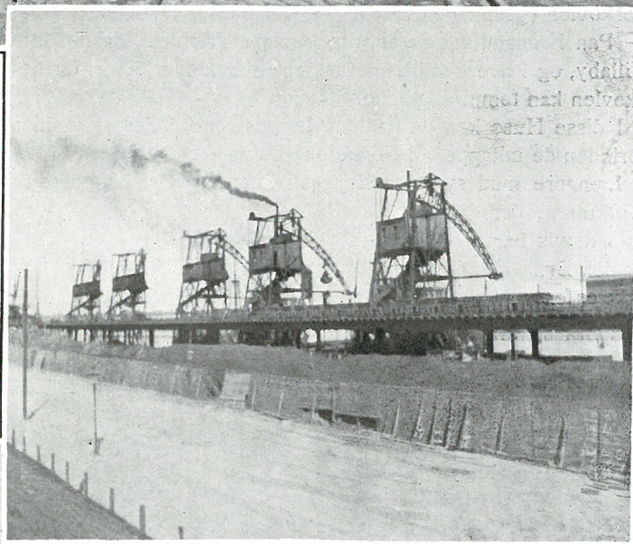
Fig. 5. Belysningsvæsenets Kraner.
