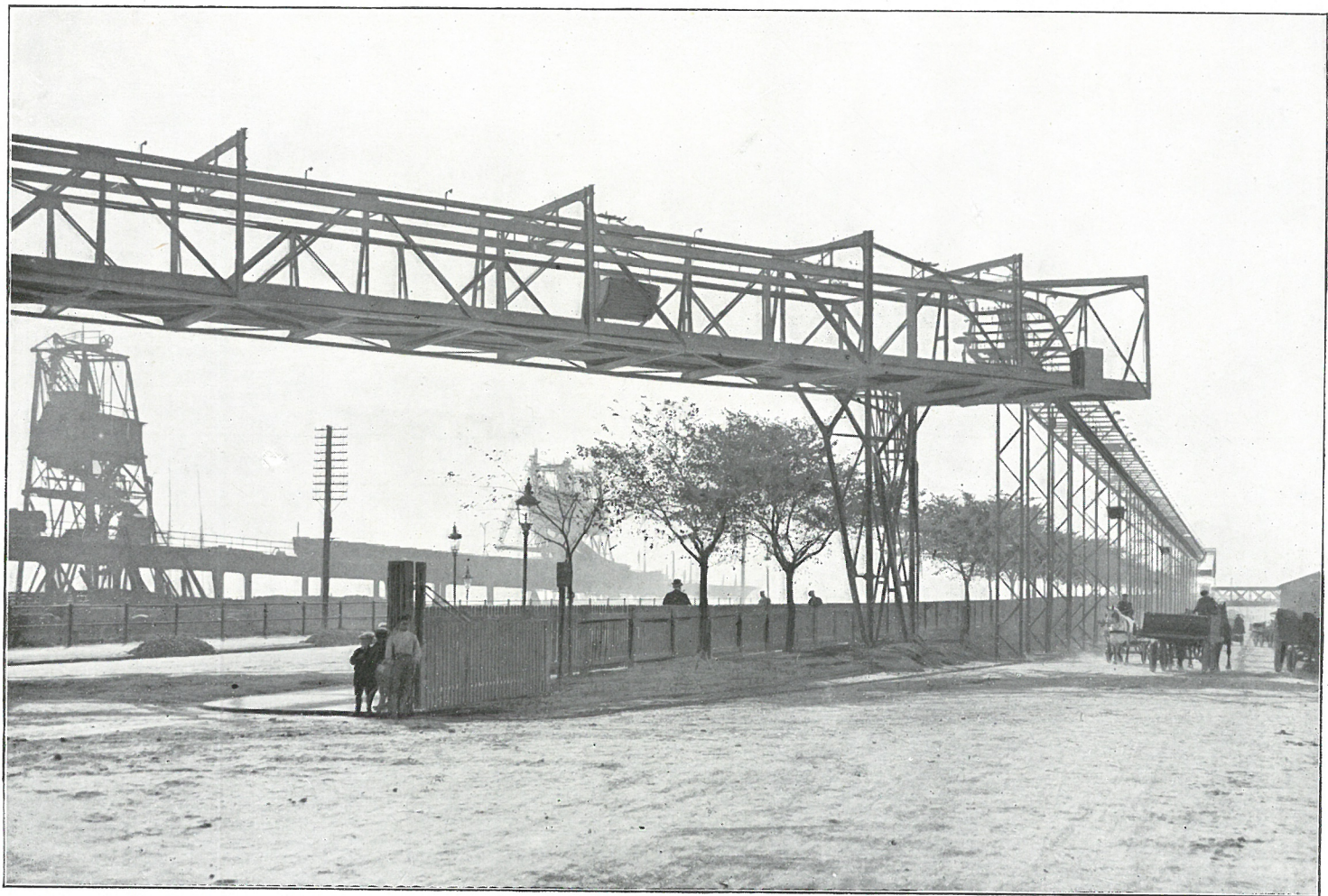
Fig. 9. Elektrohængebane paa Kalvebodbryggen.
