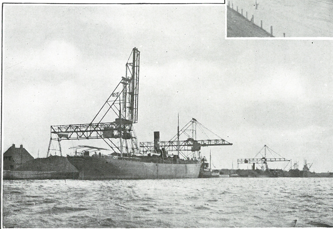
Fig. 6. Kulkraner paa Refshaleøen.
