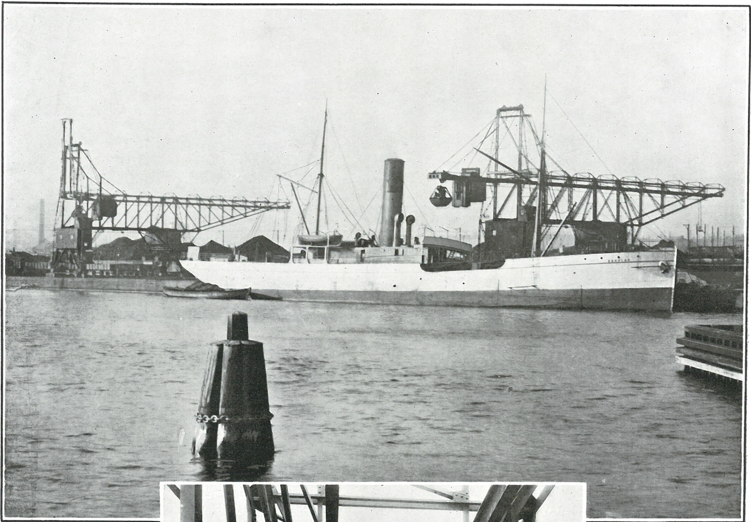
Fig. 2. Kulkran ved
