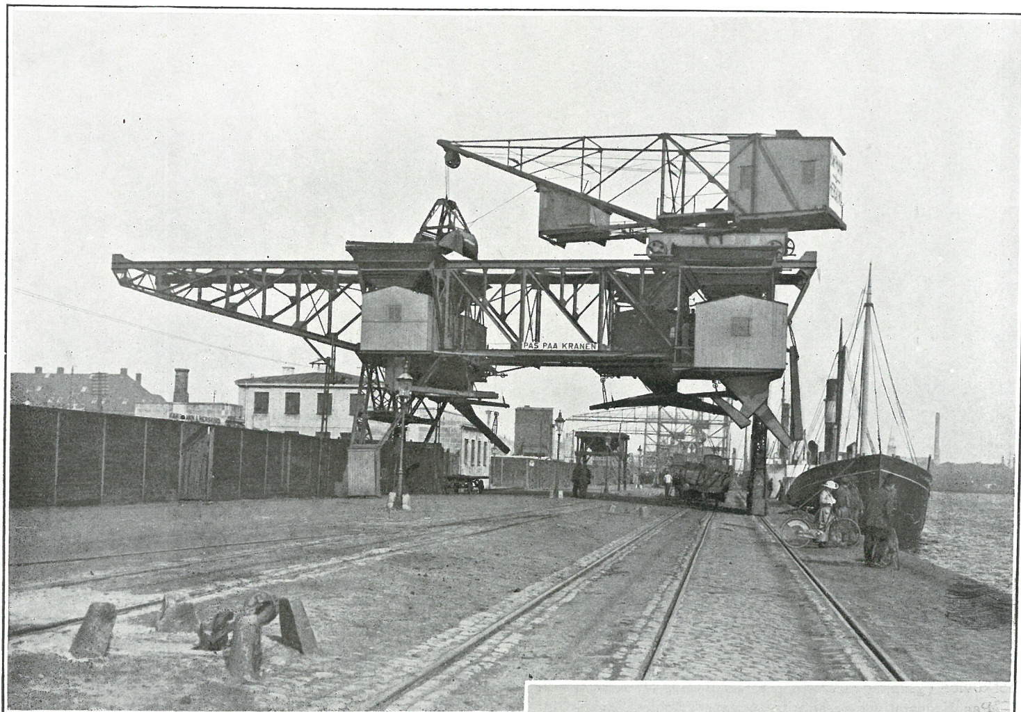
Fig. 4. Brokran.
